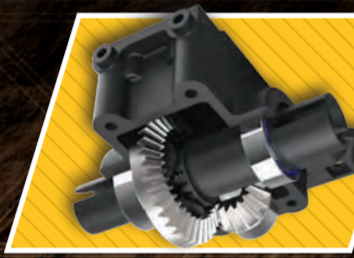
Differentials with Steel Ring and Pinion Gears Différentiels avec engrenages à anneaux et pignons en acier
