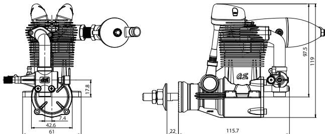
Rozměry (mm)
